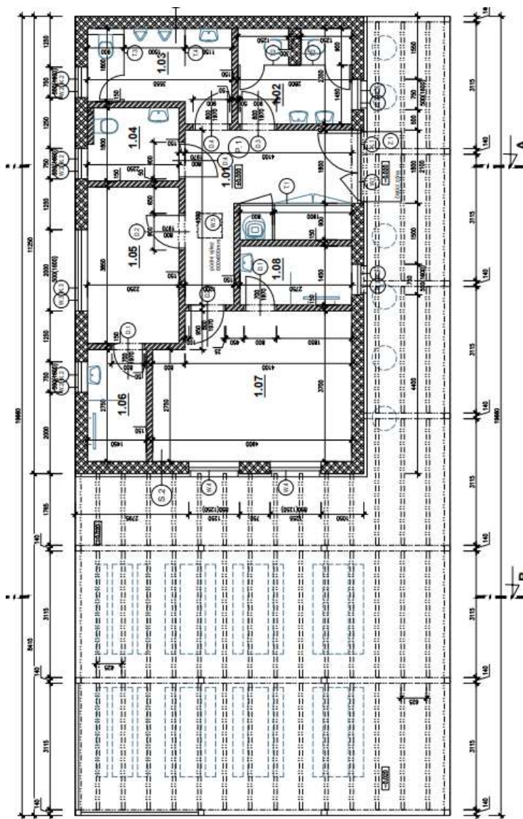
Půdorys včetně zastřešeného posezení
